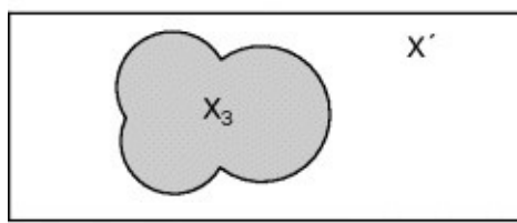
Venn diagram
